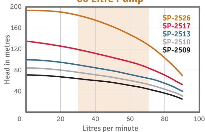
60 Litre Pump
