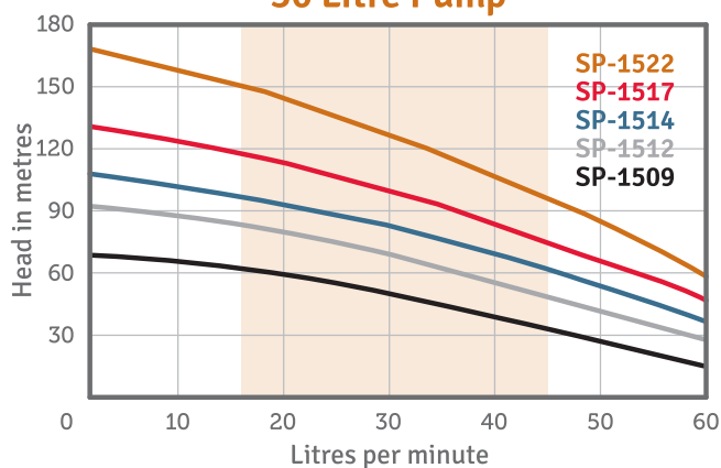
30 Litre Pump
