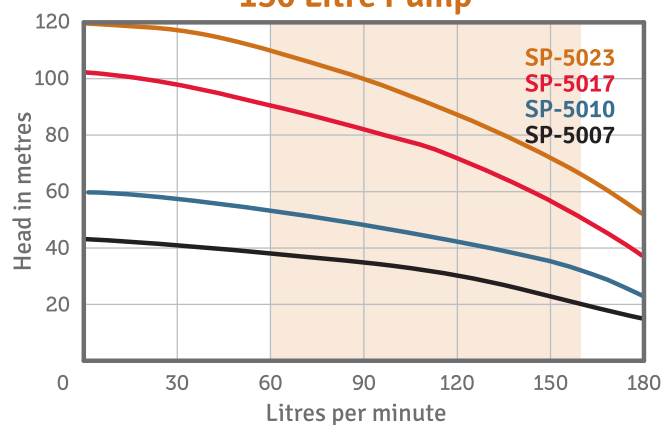
130 Litre Pump
