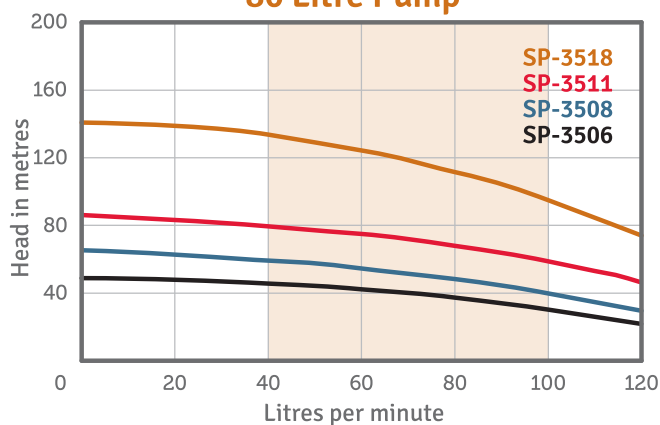
80 Litre Pump
